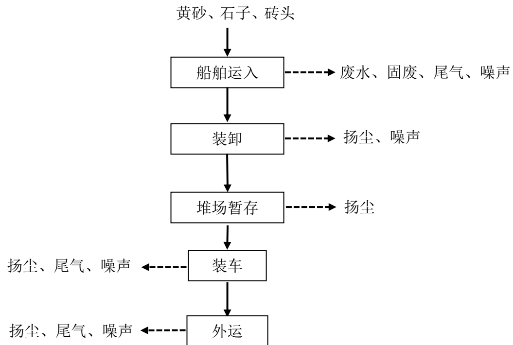
图 4-1 本项目黄砂、石子、砖头转运工作流程及产污环节图
