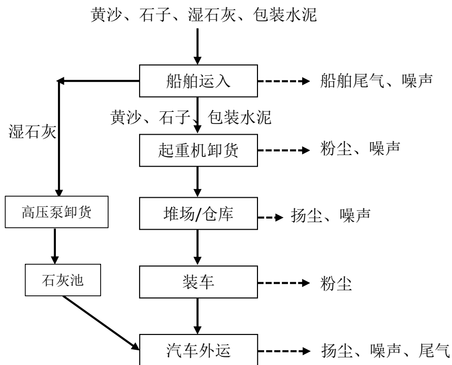
图 1-1 本项目运营期工作流程及产污环节图
