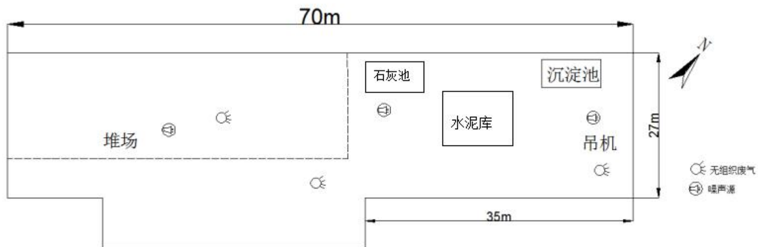
附图 3 项目平面布置图
