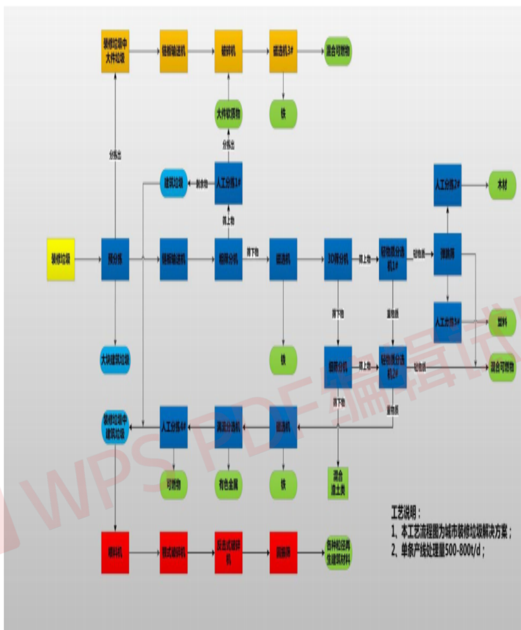
图 3.4-1 装修垃圾分选工艺流程
